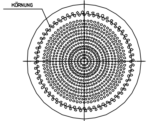
Bodenansicht
